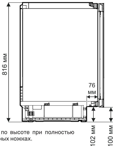
Вид сбоку
